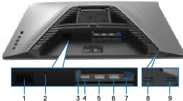
Onderaanzicht zonder monitorstandaard
